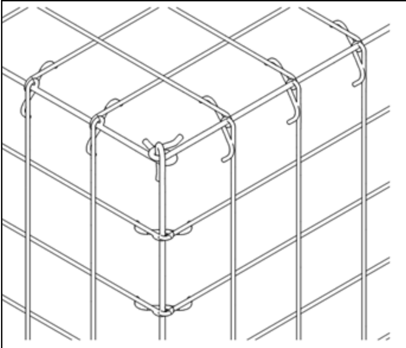
Image: tiges-goupilles correctement insérées
